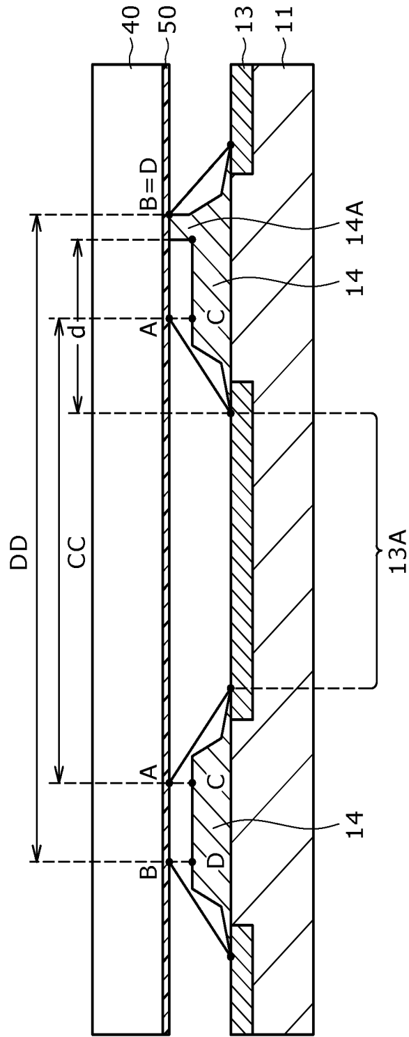
FIG. 17
